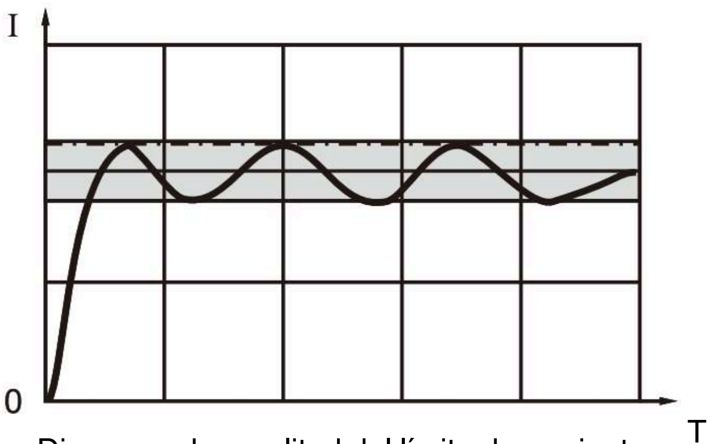
Diagrama de amplitud del límite de corriente
