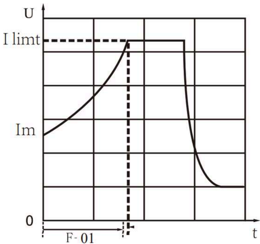
F00 = 0 Rampa de corriente
